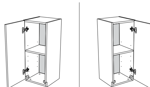
Варианты сборки
