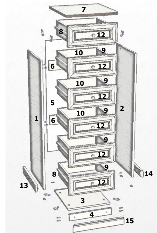
Паспорт и схема сборки
