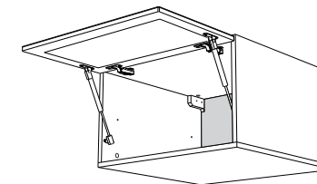
Фасад
